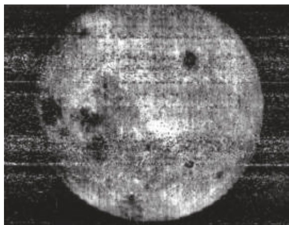
Η "αθέατη" πλευρά της Σελήνης, όπως την αποτύπωσε για πρώτη φορά το "Luna 3".
